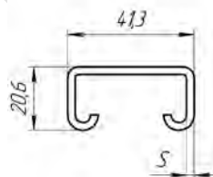
Типы и размеры Strut-профилей серии PS (длина 3 000 мм):
